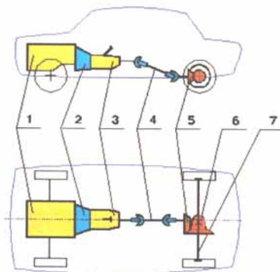
Рис. 1. Простейшая кинематическая схема автомобиля классической компоновки
